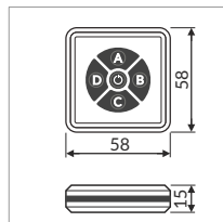
LED remote controller basic 4 channel pilot sterujący LED podstawowy 4-kanalowy
