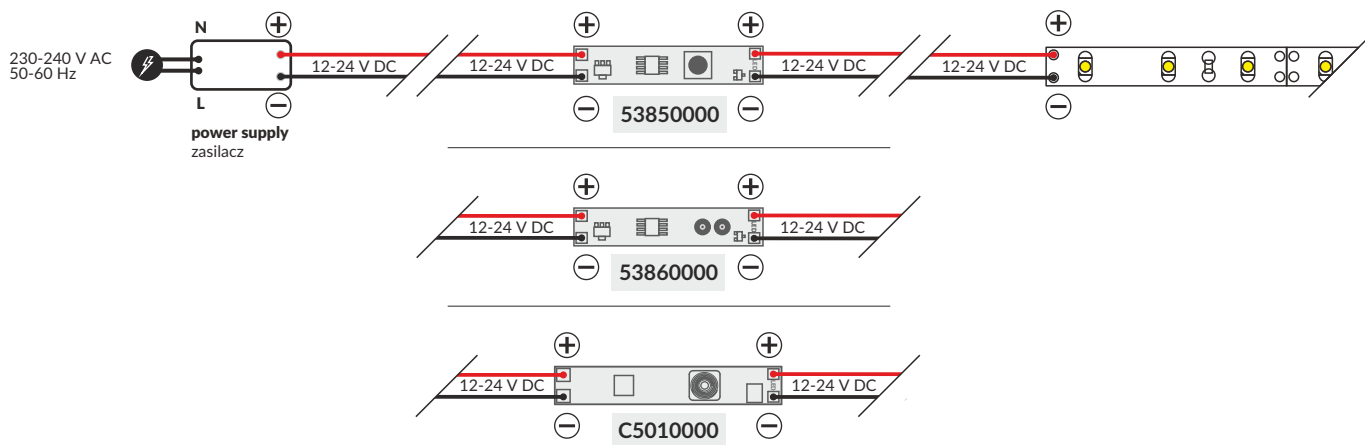
LED switch INSIDE touch dimmable włącznik LED INSIDE dotykowy ściemniający 12-24 V; 60-100 W
