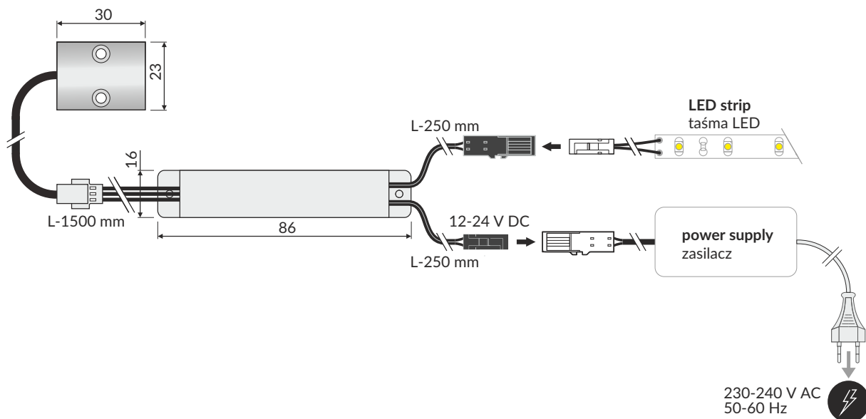
LED switch door operated sensor włącznik LED drzwiowy bezdotykowy 12-24 V; 30 W
