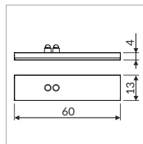
LED switch SU/GR/CO touchless dimmable włącznik LED SU/GR/CO bezdotykowy ściemniający 12-24 V; 60-100 W
