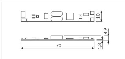
LED receiver basic 1 channel moduł sterujący LED podstawowy 1-kanalowy 12-24 V; 60-100 W
