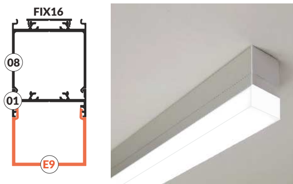
variant 15 - ceiling FIX16-08-01-E9 variant 15 - sufitowy FIX16-08-01-E9
