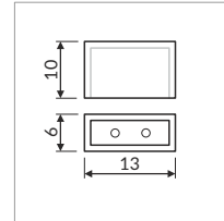
ending for silicone housing for 8 mm LED strip zaślepka do osłony silikonowej do taśmy LED 8 mm
