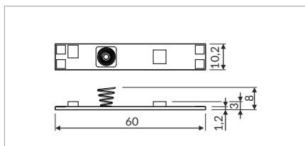
LED switch INSIDE touch dimmable włącznik LED INSIDE dotykowy ściemniający 12-24 V; 60-100 W
