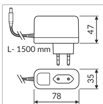
18 W 12 V / 100-240 V AC adapter / zasilacz wtyczkowy 15820002
