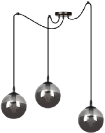
937/3 GIGI 3 BL/GRAFIT wys. max 200 cm 3 x E27 max 40 W
