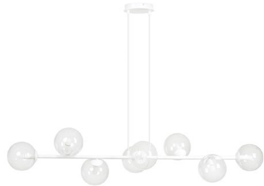
877/8 ROSSI 8 WH/TRANSPARENT wys. max 100 cm szer. 130 cm 8 x E14 max 40 W
