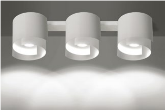
925/3 STYLE 3 WHITE wys. 14 cm szer. 63 cm 3 x GU-10 max 30 W
