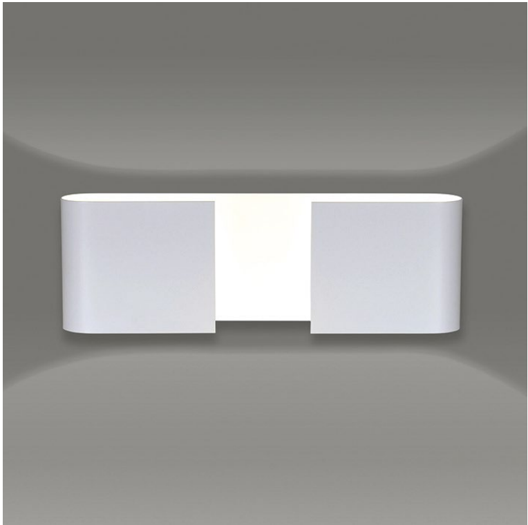
933/1 DUO WHITE wys. 12 cm szer. 36 cm 2 x G9 max 20 W
